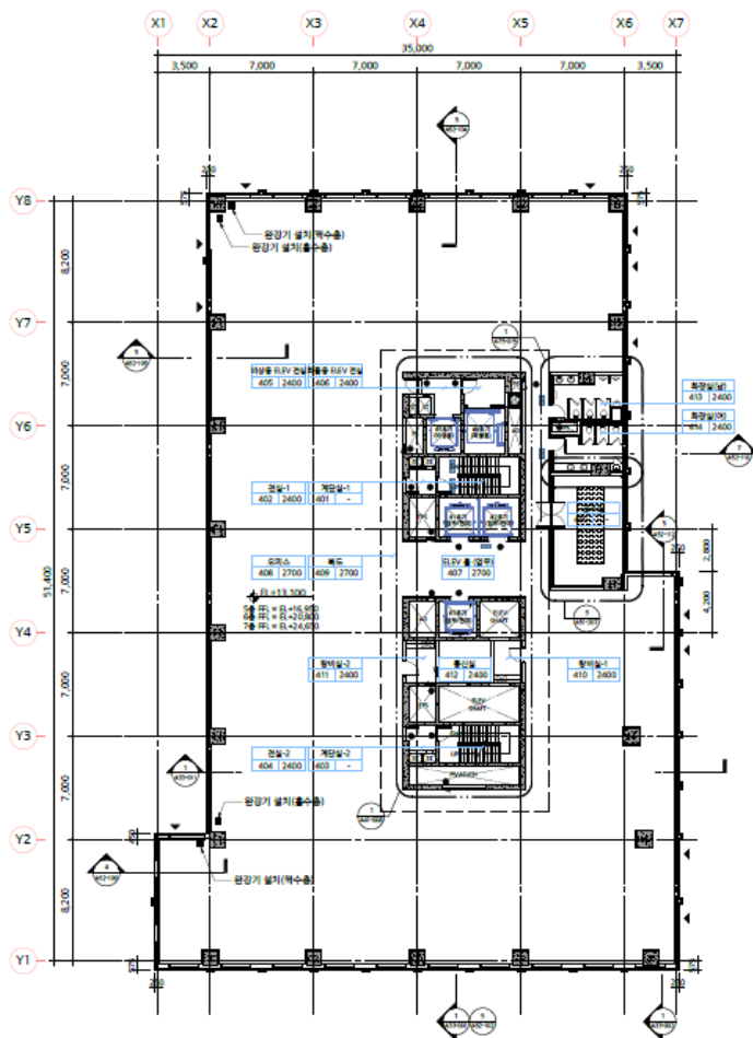
평면도 (7층)
